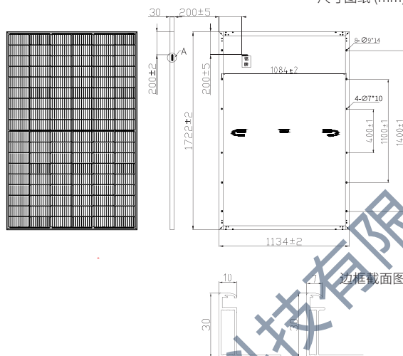
尺寸图纸 (mm)
